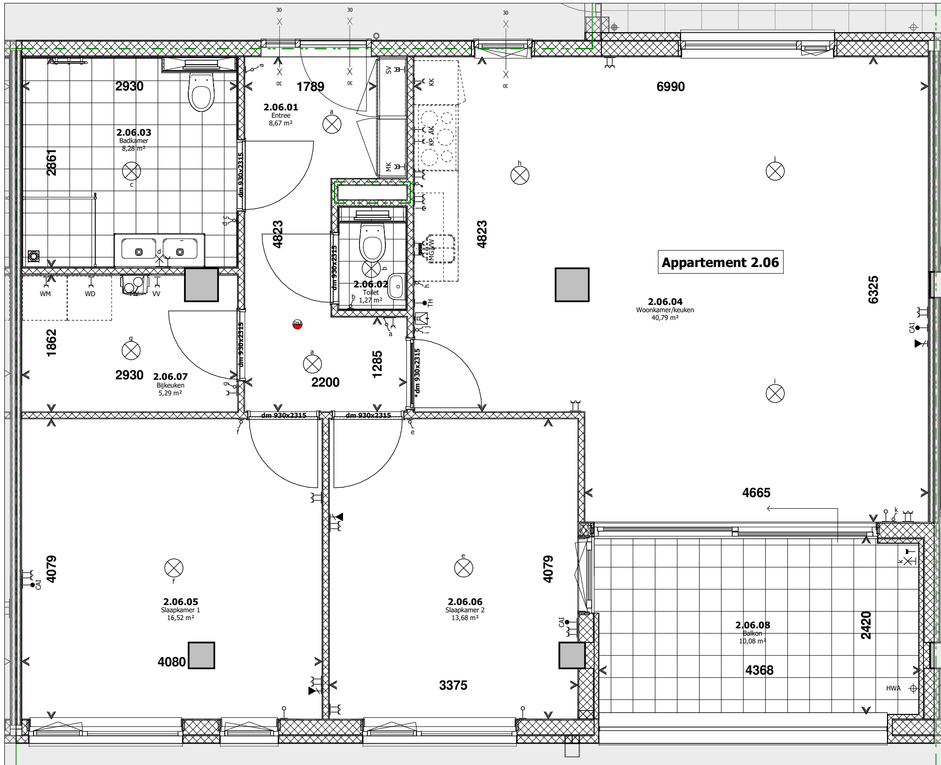
2e verdieping
