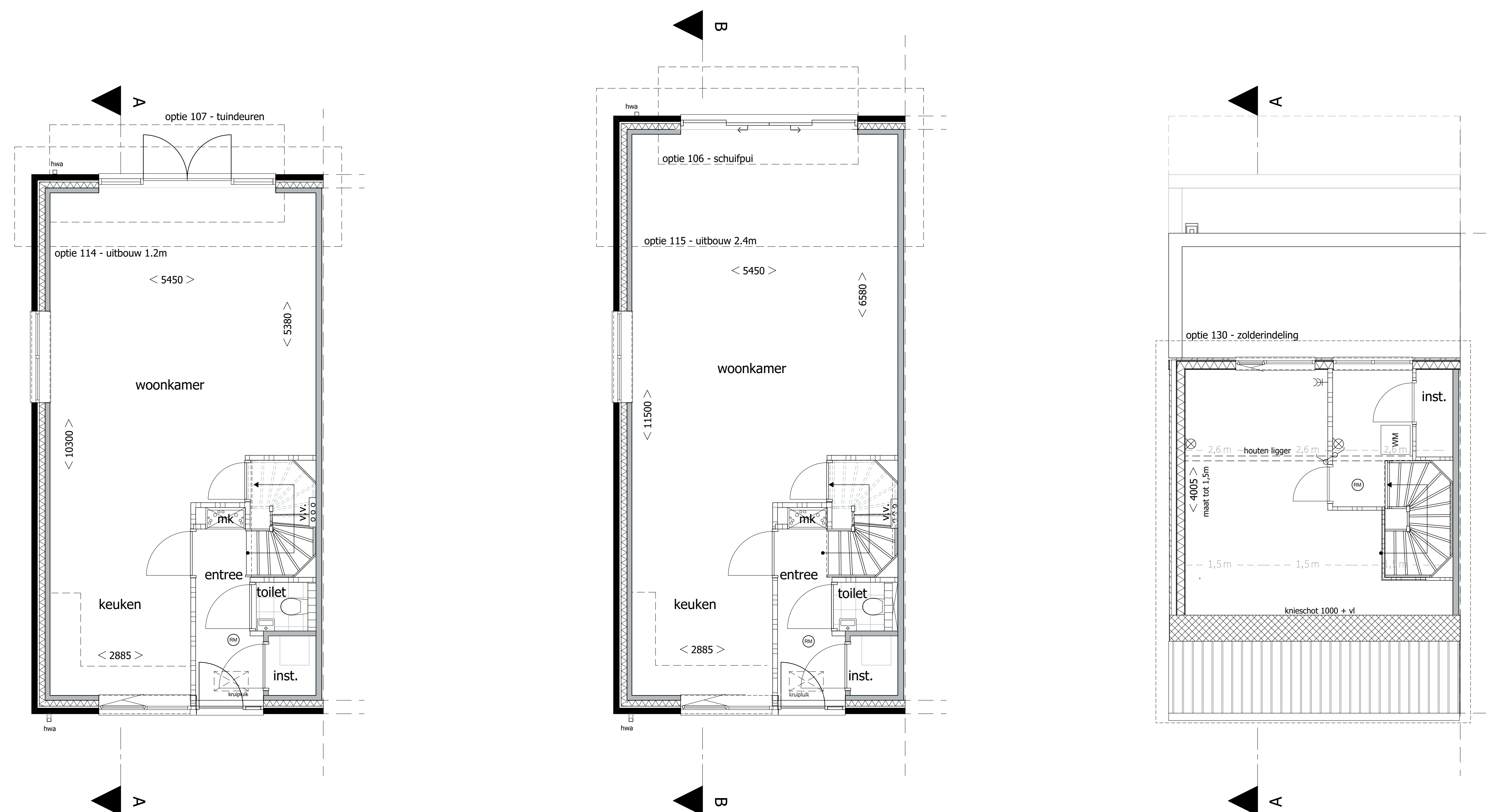
Begane grond type E4 Opties E5 gelijkwaardig Bouwnummers 80, 83
