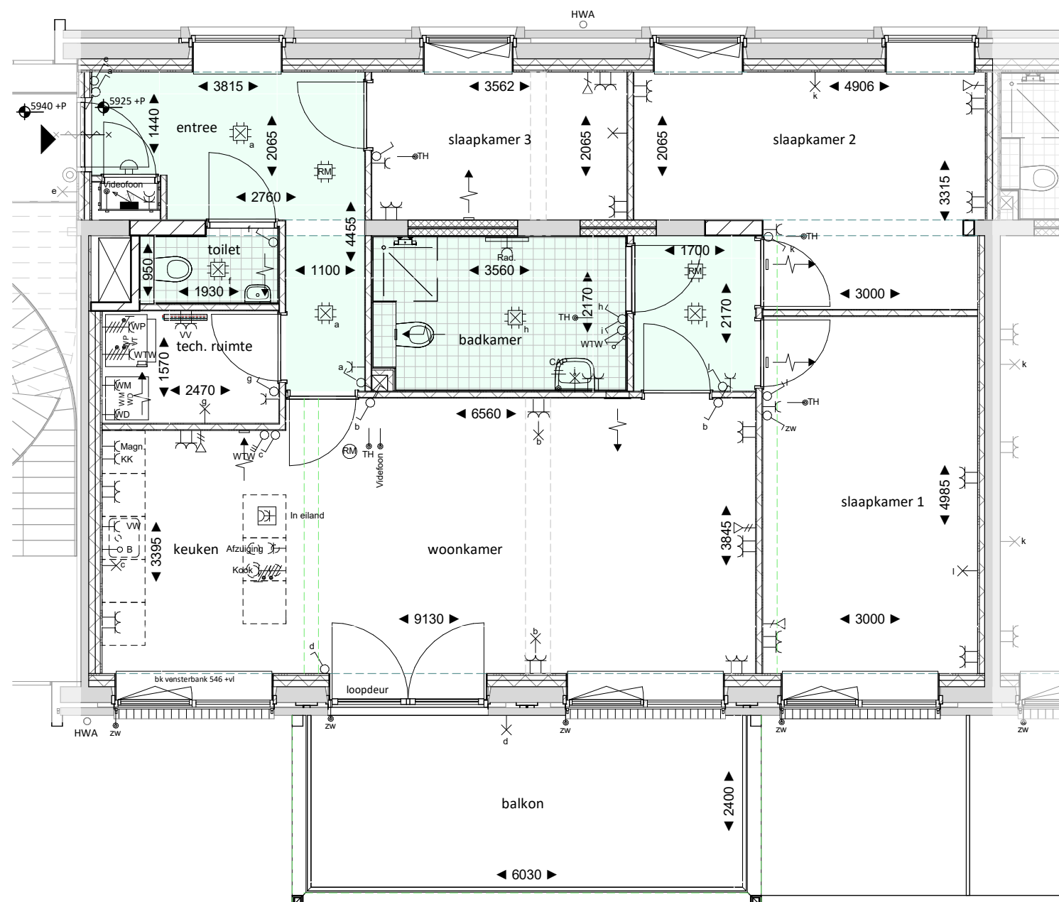
01 eerste verdieping
