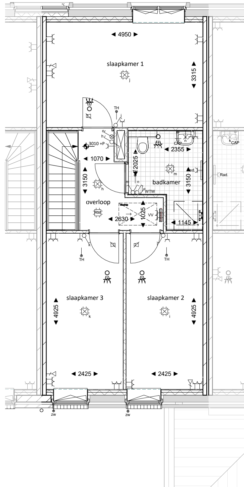
01 eerste verdieping
