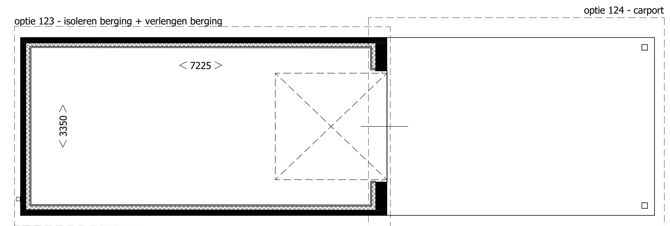
Berging plattegrond Bouwnummer 51 & 52 (gespiegeld)
