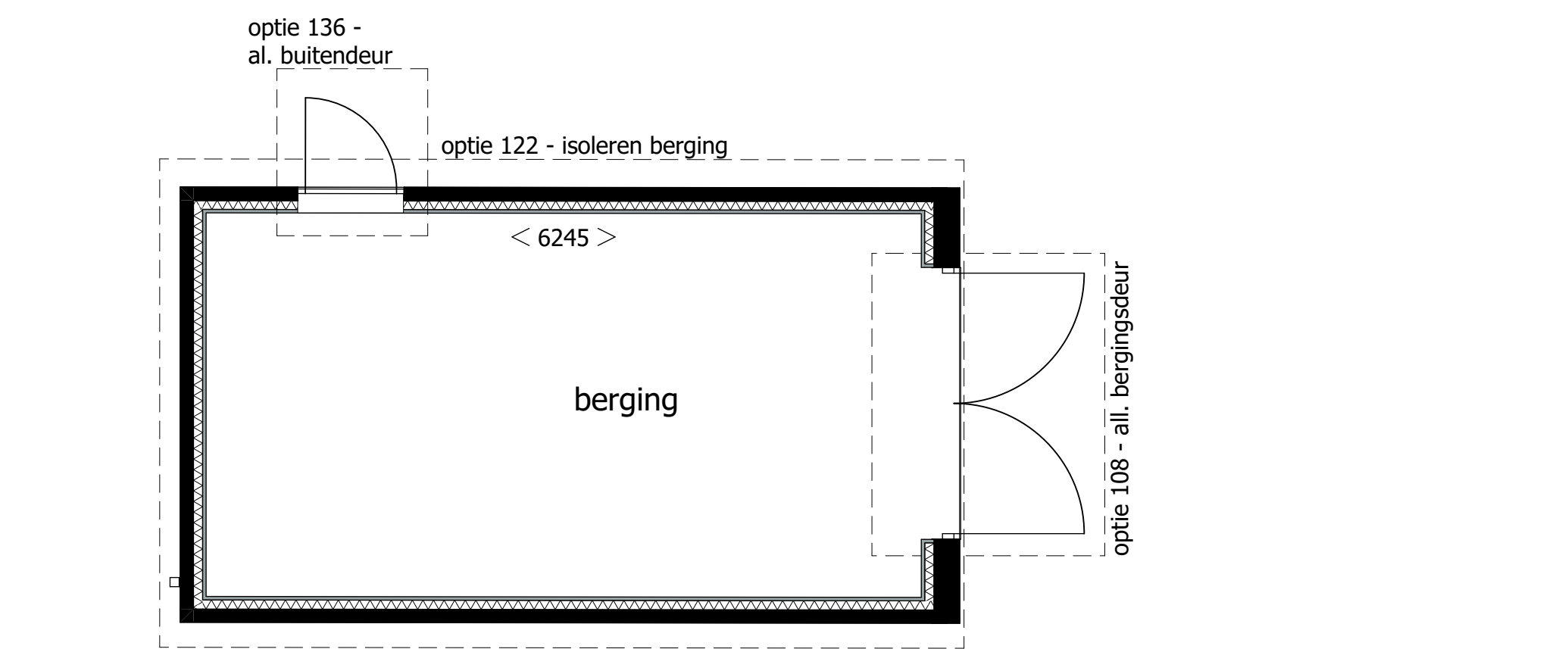
Begane grond type A1 Bouwnummer 51 & 52 (gespiegeld)
