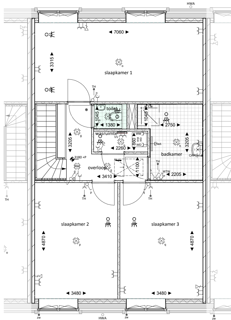
01 eerste verdieping 1 : 75
