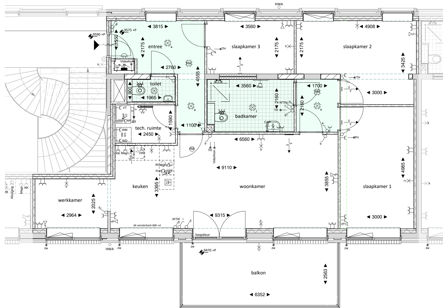
02 tweede verdieping
